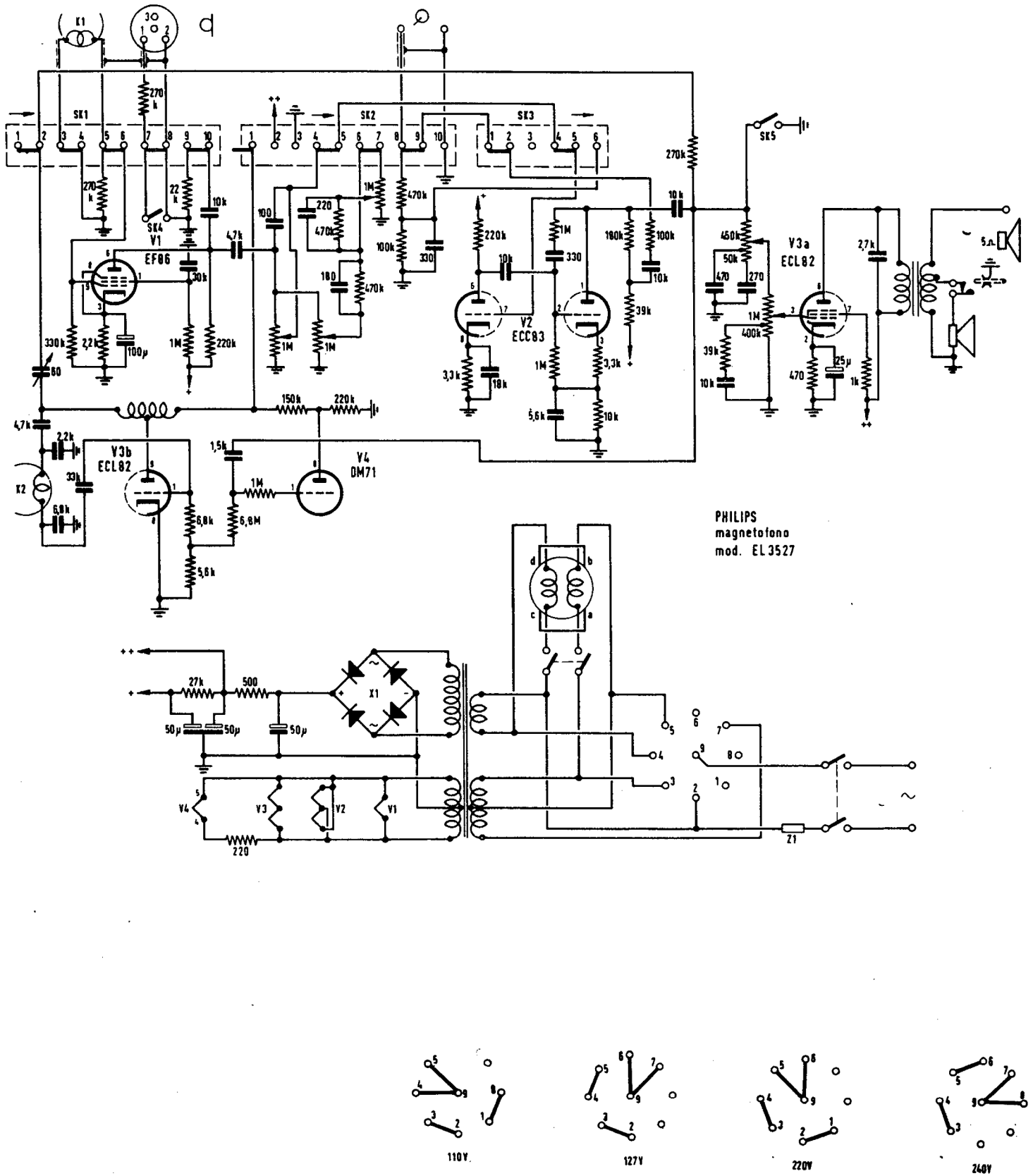
Schema elettrico del magnetofono, PHILIPS mod. EL3527
